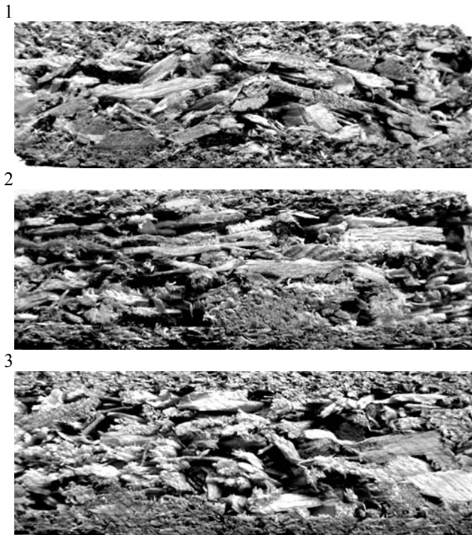
Fig. 2. Cross-sections of tested particleboards Rys. 2. Przekroje badanych płyt wiórowych
